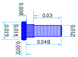
DETALLE DE ESPARRAGO
