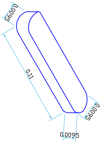
DETALLE DE CUÑA
