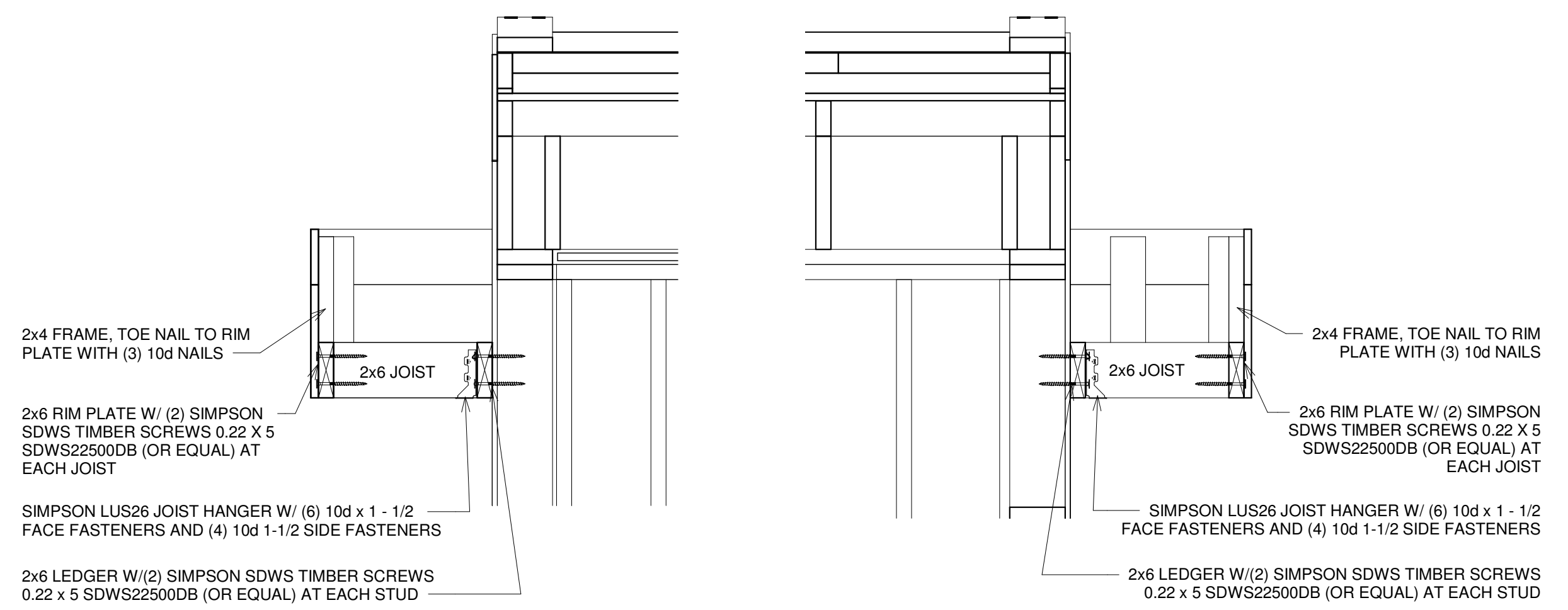
2 PARAPET LEFT SCALE: 1" = 1'-0"
