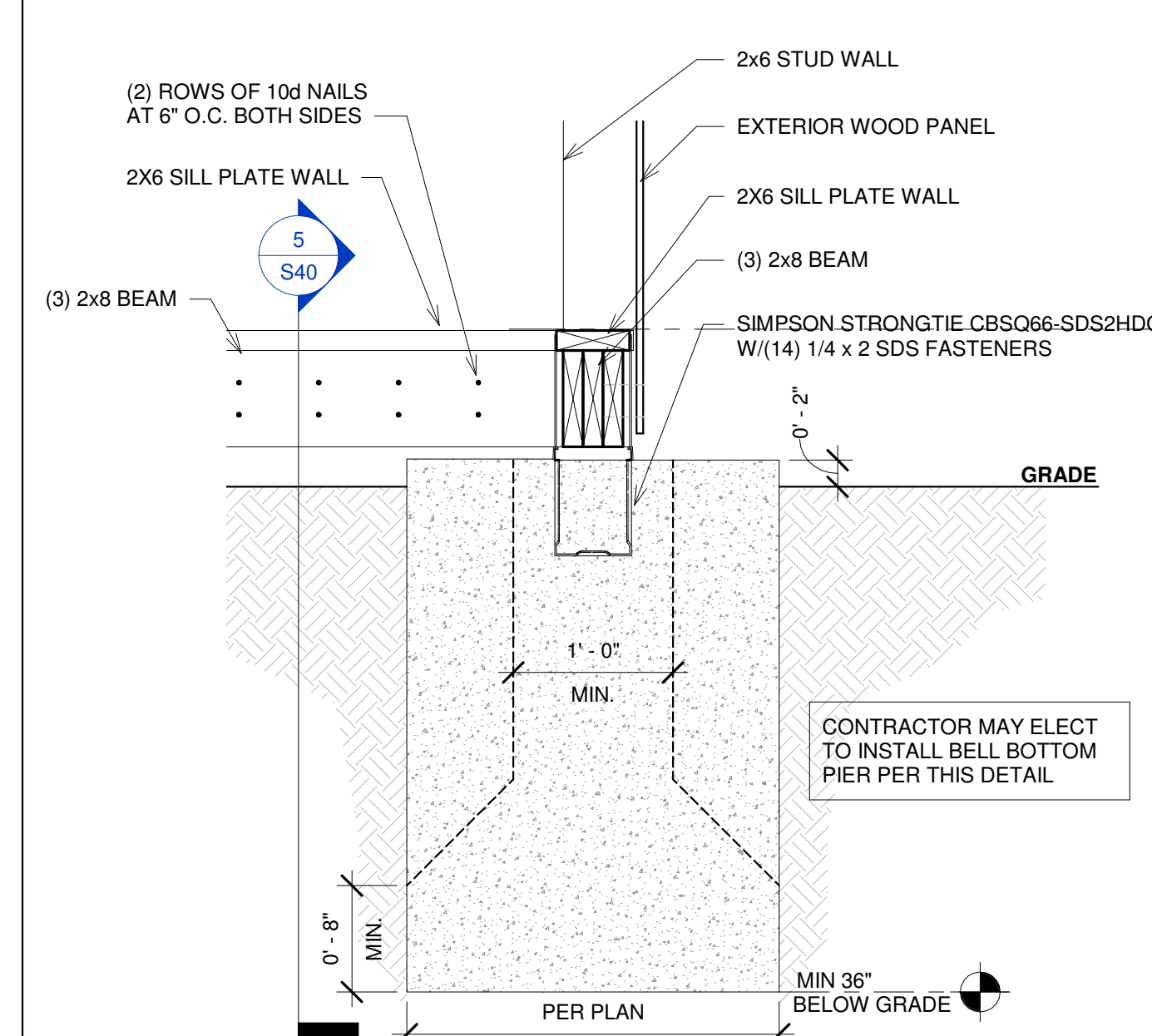
7B SECTION 7B SCALE: 1" = 1'-0"
