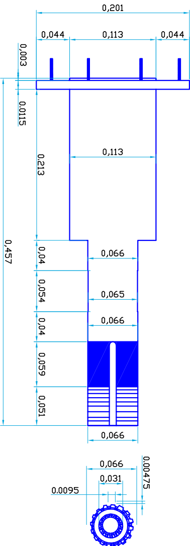
PLANTA EJE
