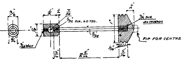
BUCKET & ROD
